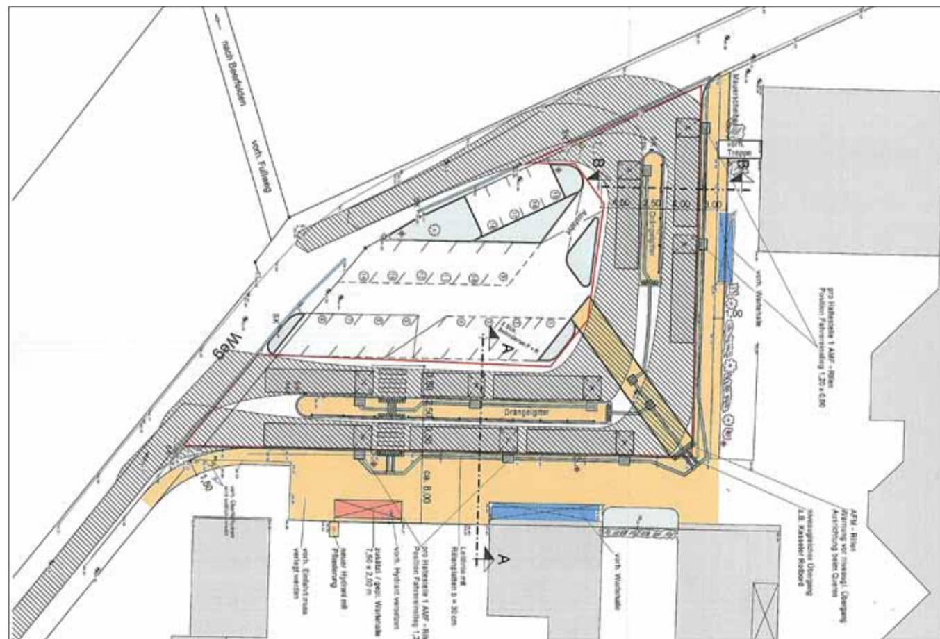
Skizze des neuen Busbahnhofs der Oberzent-Schule Beerfelden, erstellt vom durchführenden Ingenieurbüro Krimmelbein.
